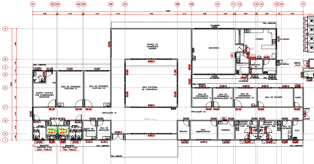
01 CENTRO DE ATENÇÃO PSICOSSOCIAL I PLANTA PAVIMENTO TÉRREO ESCALA 1/10
