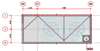
02 CENTRO DE ATENÇÃO PSICOSSOCIAL I, II, AD E I PLANTA DE COBERTURA ESCALA 1/10
